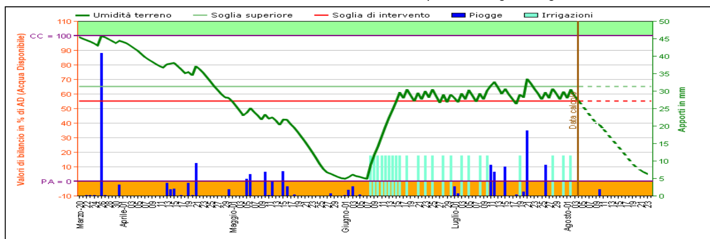
Grafico storico indicante l'andamento del bilancio idrico nella presente stagione irrigua
